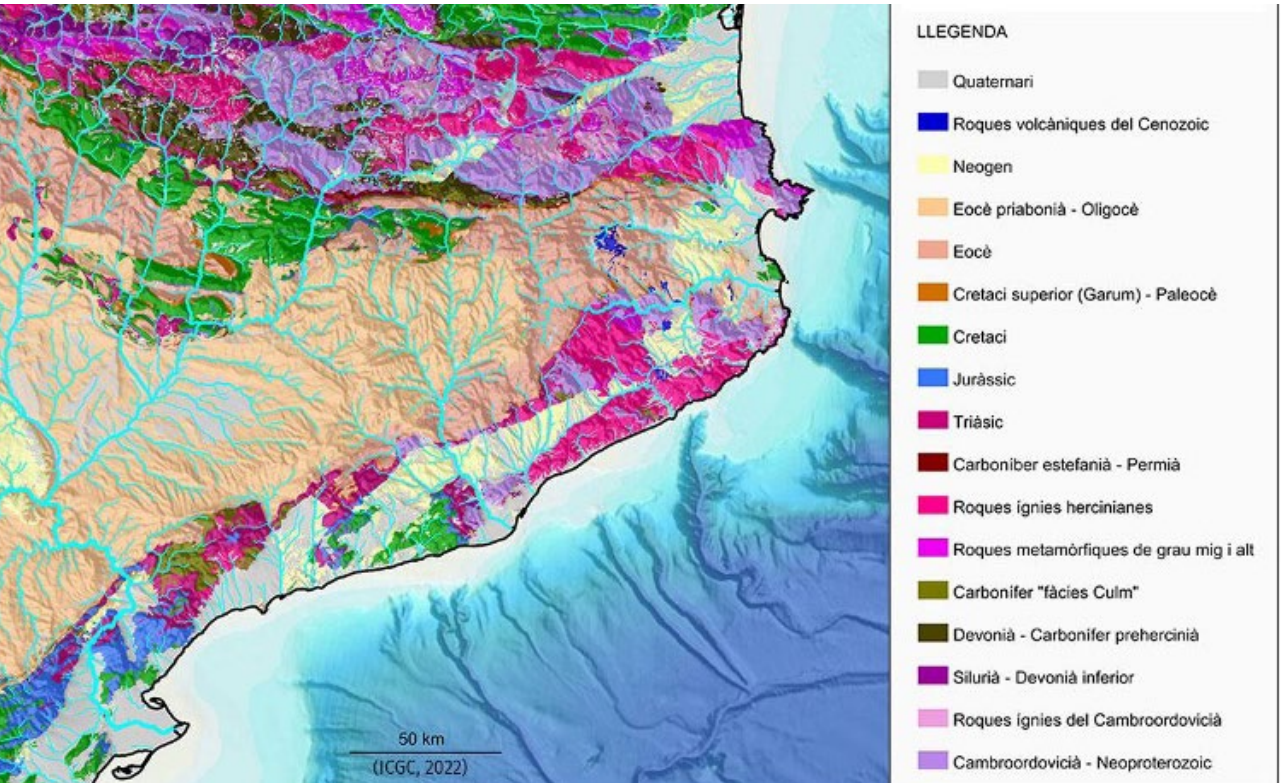
Mapa de contextualització geològica de Catalunya i els seus entorns derivat del Mapa Estructural de Catalunya 1:250.000 (Font: ICGC)
